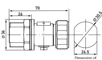
P8AX_-716/MF
