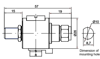
P8AX_-F/MF
