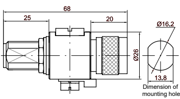
P8AX_-N/MF
